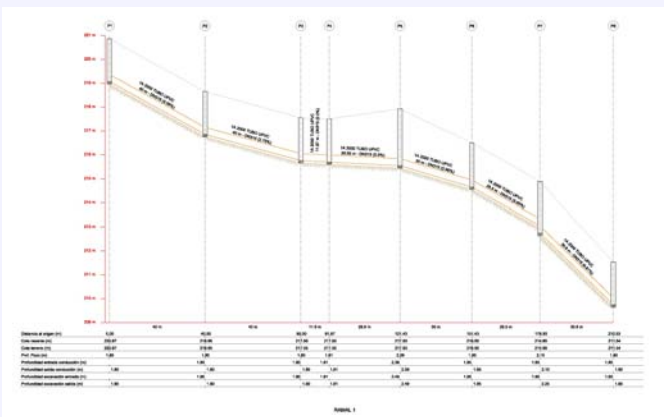
Sección longitudinal .
