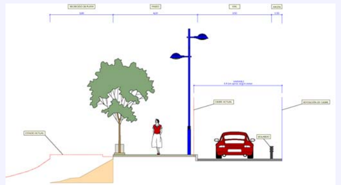
Sección tipo.
