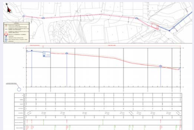
Perfil longitudinal
