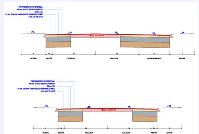
Secciones tipo.
